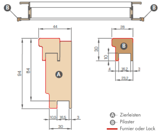
Schnitt Z
