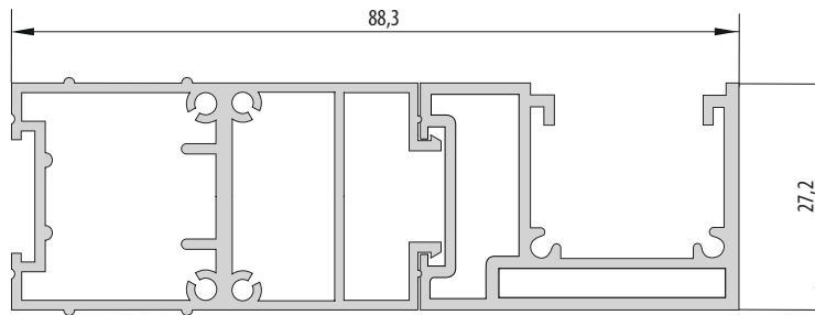
Monoblock-Führungsschienen SOLID
